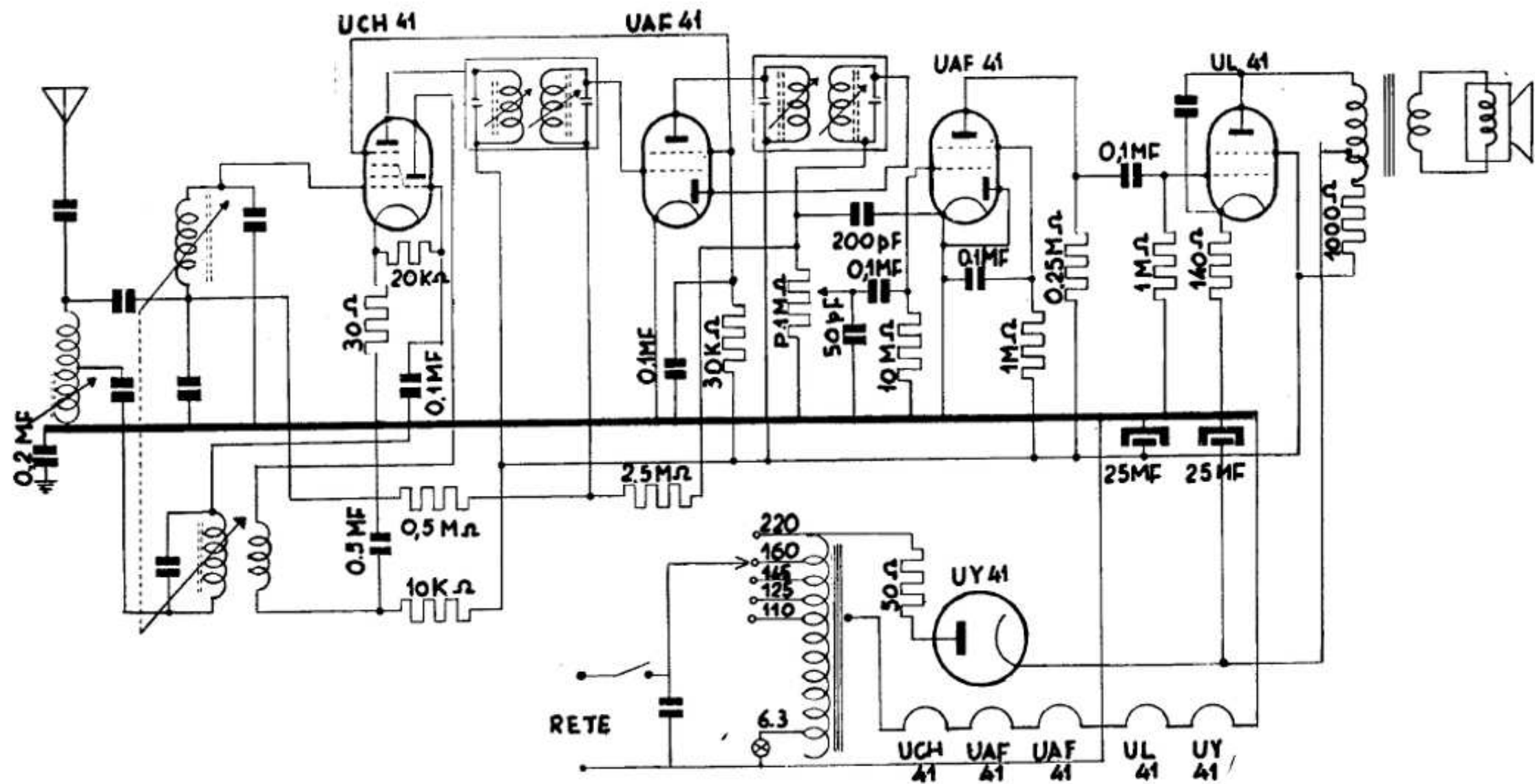
ALTAR - Mod. RM 9 (AR 48). Onde medie da 180 a 590 metri. Media frequenza 467 kc/s. Potenza d'uscita indistorta 1,5 watt. Consumo 30 watt.
